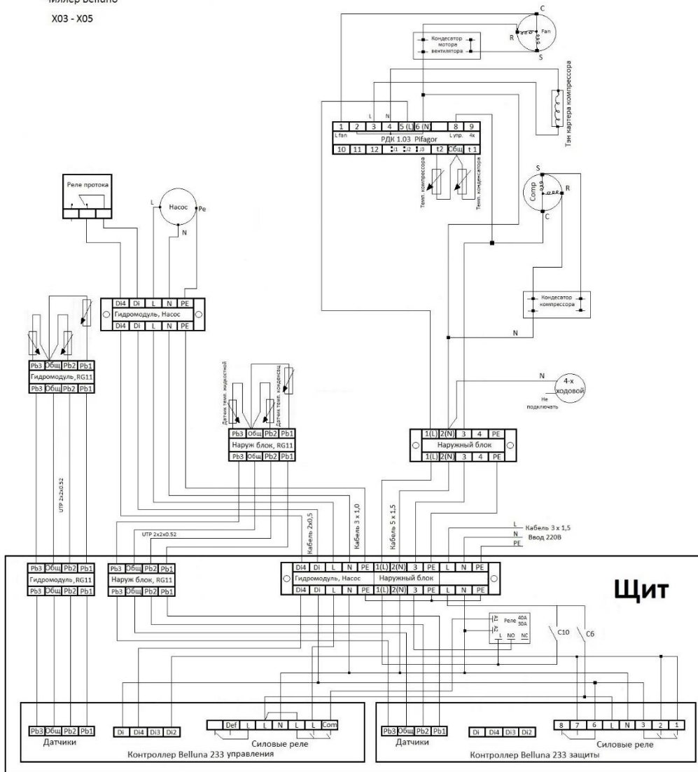
Рис 2. Электрическая схема подключения холодильной машины
